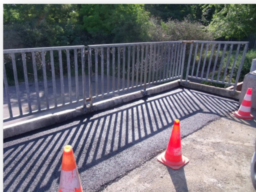
Reprise des enrobés en haut de quai
