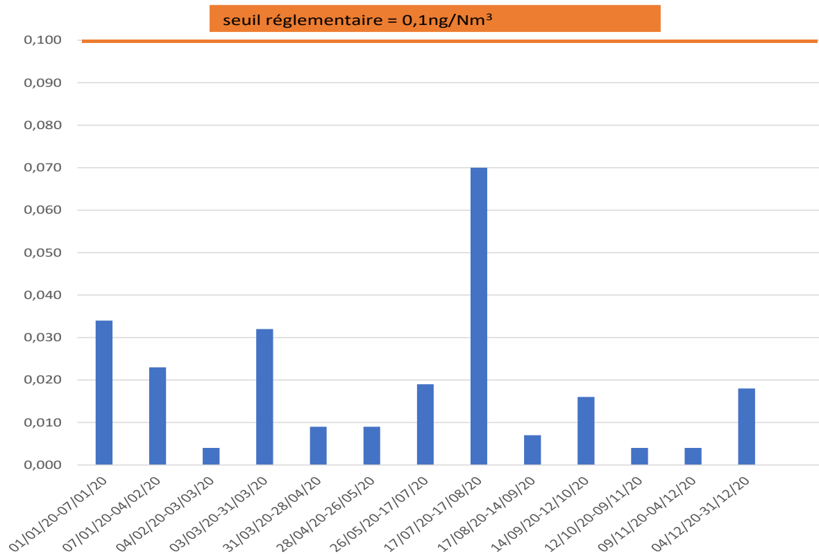
Contrôle semi-continu des dioxines 2020- concentration en ng/Nm 3
